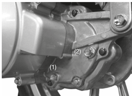
(1) Vite di drenaggio (2) Vite di ispezione
